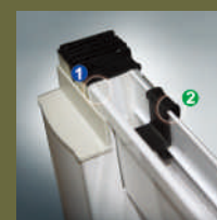
1. 內框防水布 2. 內框防晃動滑塊
