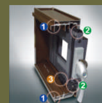
1. 多空心結構外框設計 2. 內框上下側阻風板 3. 外框止水阻風塊
